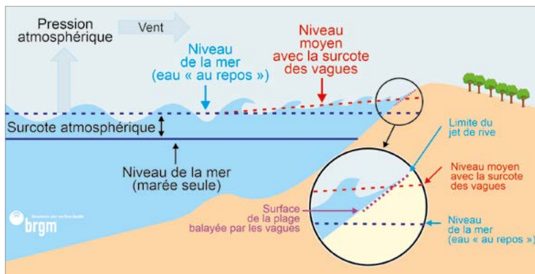
fig. les processus qui déterminent les niveaux de la mer et la submersion
