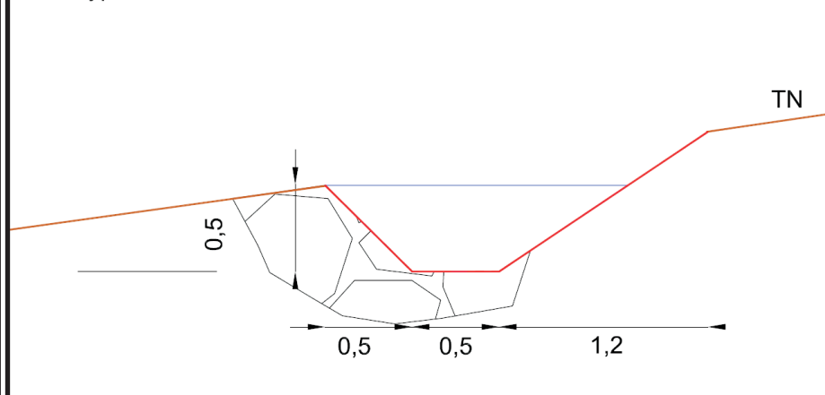
Profil type du ruisseau dévié
