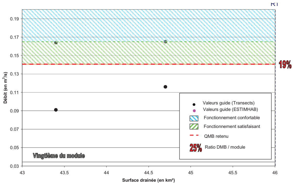
Figure 8 : Débit Minimum Biologique du bassin du Riu Ferrer
