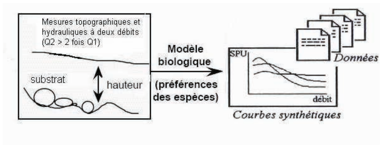
Figure3 : Schéma de présentation de la méthode ESTIMHAB
